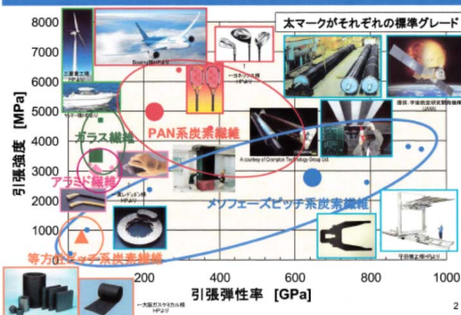
各種高性能繊維の物性とそれらを使用したCFRPの用途例
