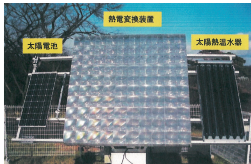
追尾集光型太陽エネルギー利用システムの開発
